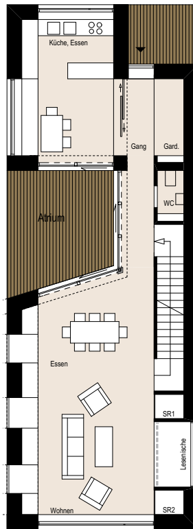
Erdgeschoß
